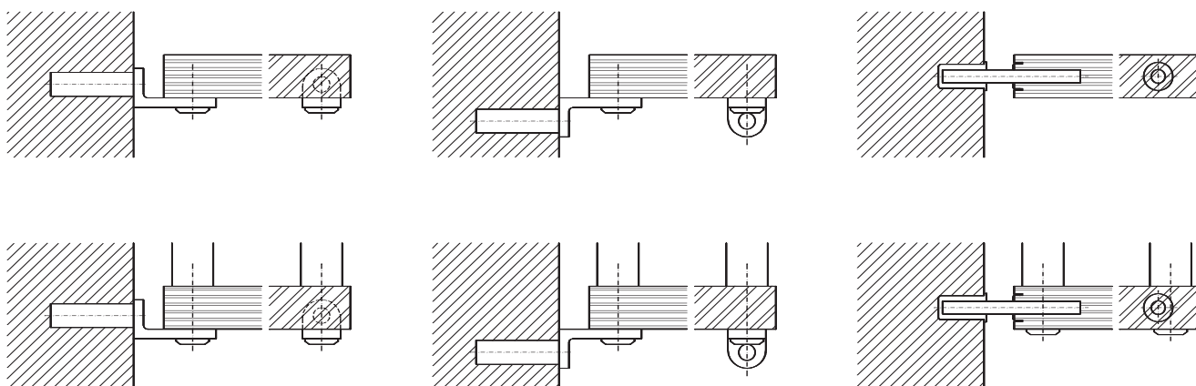
Wandanker: Winkel
